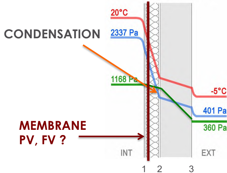
Cas 1 : isolation intérieure
