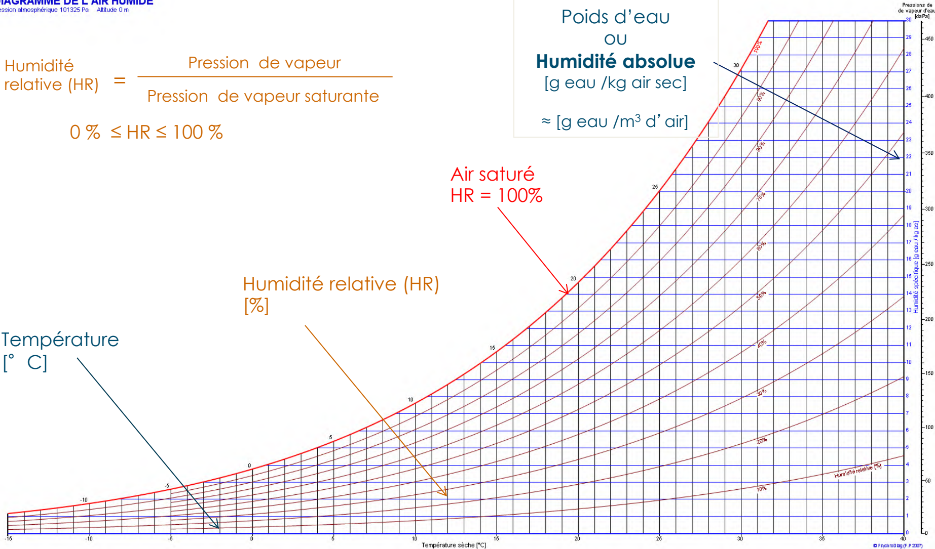
DIAGRAMME DE L'AIR HUMIDE Pression atmosphérique 101325 Pa Altitude 0 m
